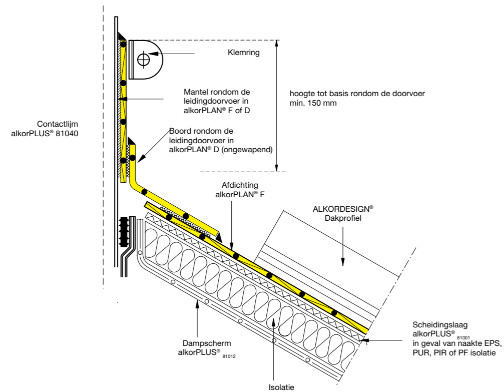
Leidingdoorvoer
