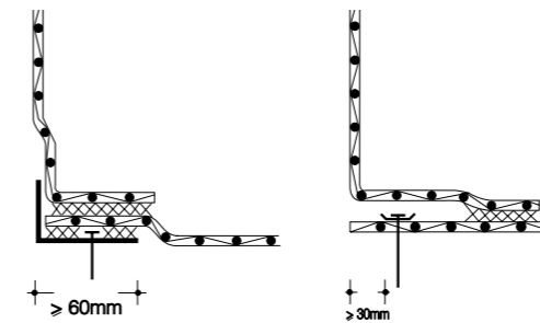
Fig. 3: Kimfixatie met alkorPLUS® folieplaat
