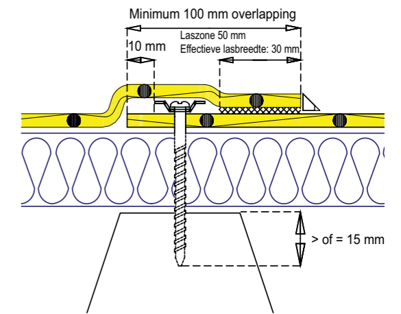
Fig.1: Mechanische bevestiging en overlapping van de dakbaan
