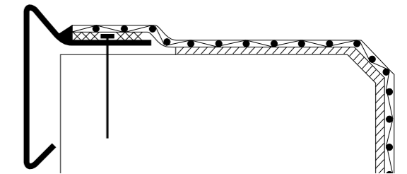
Fig. 4: Volvlakkige verlijming
