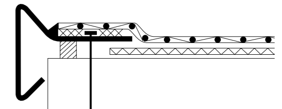
Fig. 5: Gebruik van een winddichtingsband alkorPLUS® 81058
